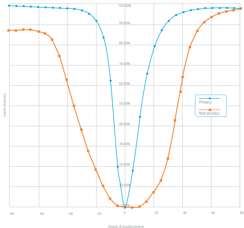
Figura 3a. Aree di visualizzazione privacy e non privacy – HP EliteBook 840 G3/G4, 1040 G3
