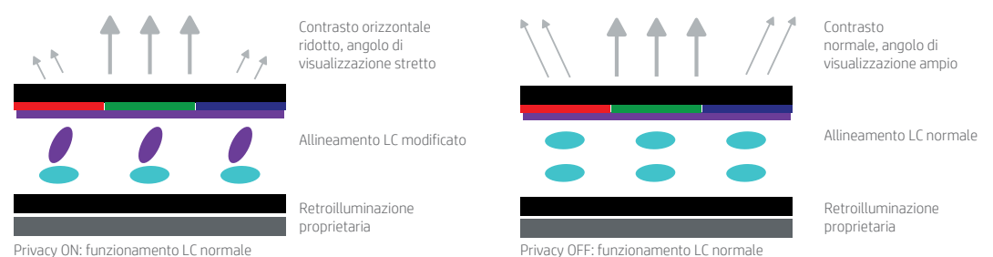
Figura 1b. Funzione di illuminazione – HP EliteBook x360 1030 G2
