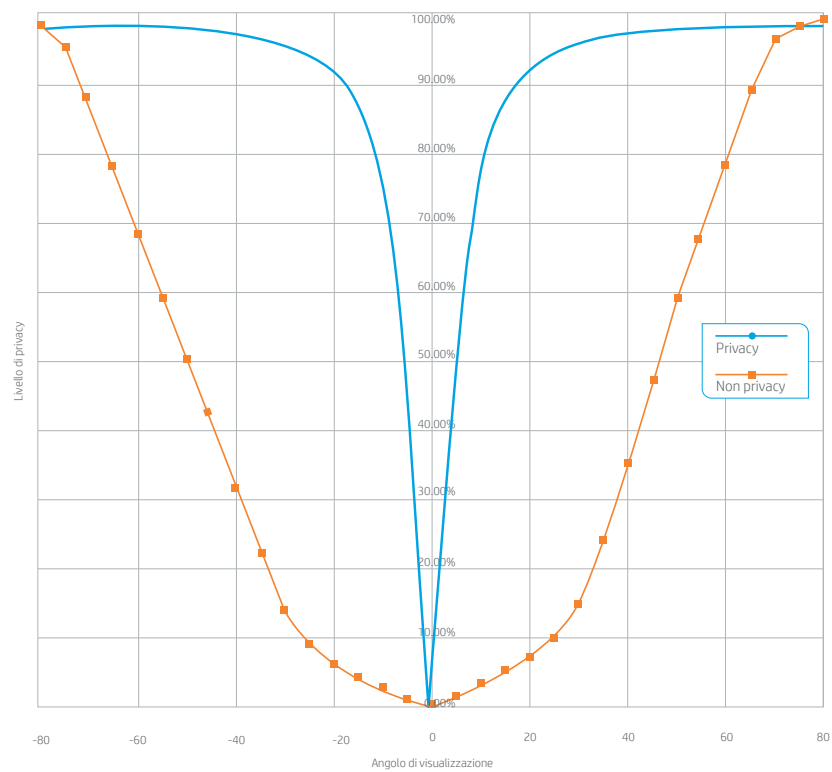
Figura 3b. Aree di visualizzazione privacy e non privacy – HP EliteBook 840 G3/G4, 1040 G3
